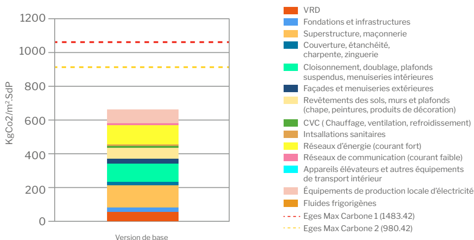
Impact carbone sur la phase de construction (Eges pce)
