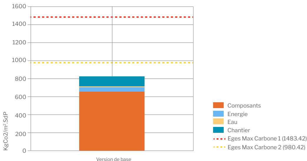
Impact carbone sur tout le cycle de vie (Eges)
