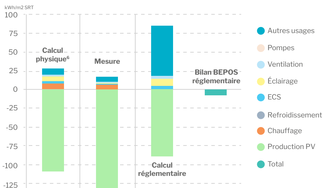
Bilan des consommations tous usages et de la production photovoltaïque du bâtiment LowCal, année 2016-2017
