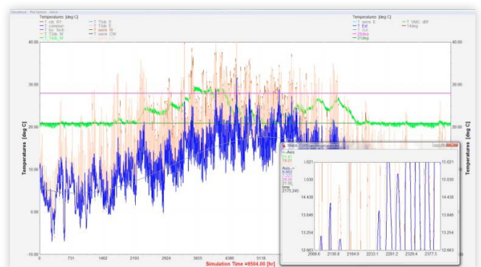
Simulation TRNSys pour le confort d'été et les besoins de chauffage
