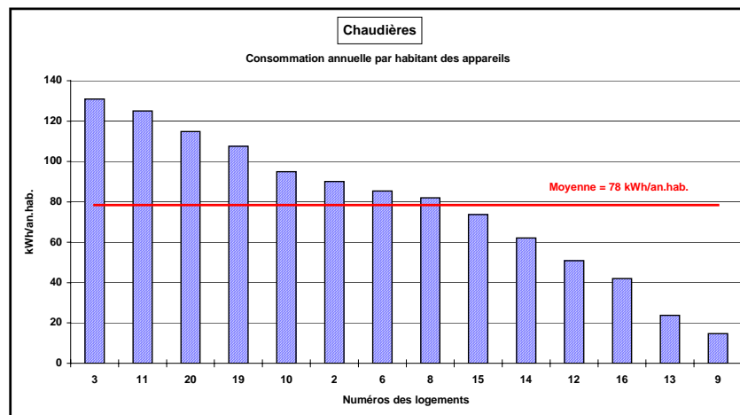
Figure 1.2 : consommation par habitant et par an des chaudières gaz murales
