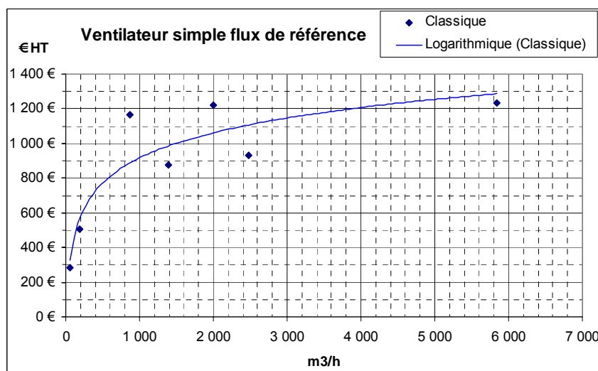
Graphique 2 : prix de référence des ventilateurs simple flux classiques en fonction du débit de pointe
